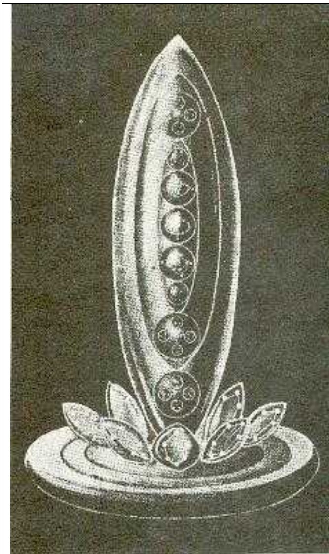
Estructura atómica del LITIO:
