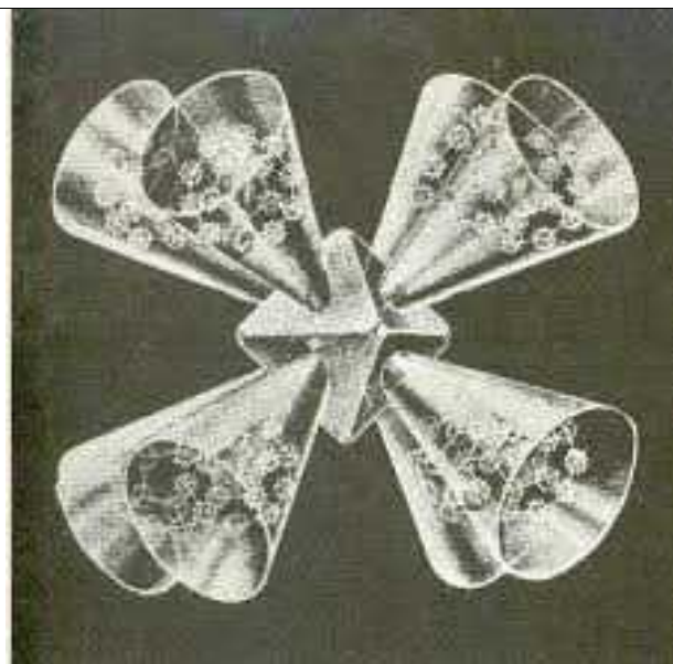
Estructura atómica del HIERRO;
